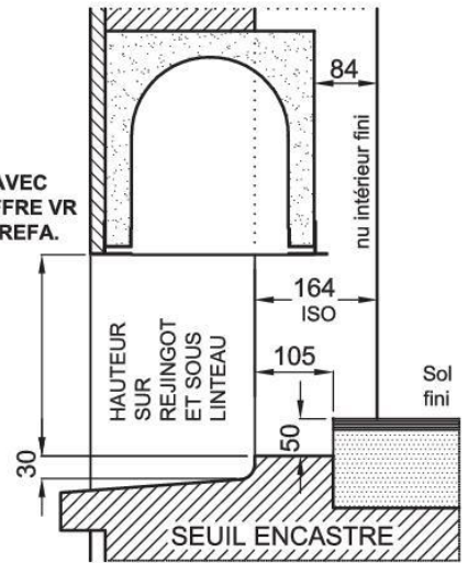
COUPES VERTICALES
