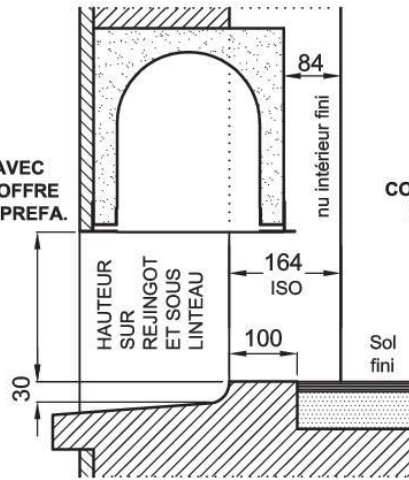
COUPES VERTICALES
